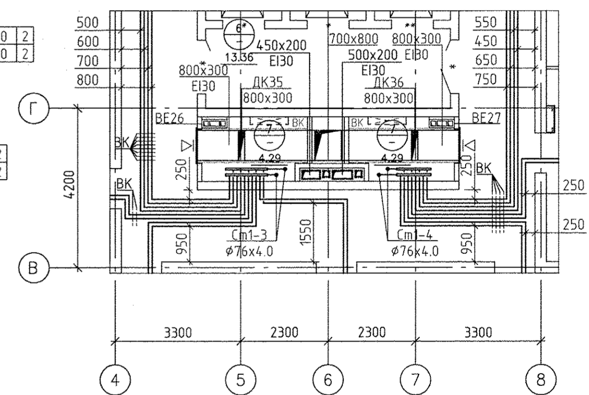
Фрагмент плана 19 этажа
