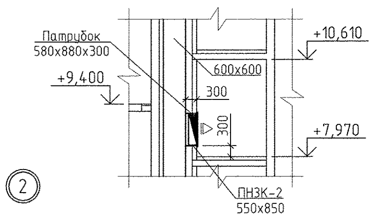
Разрез 1-1
